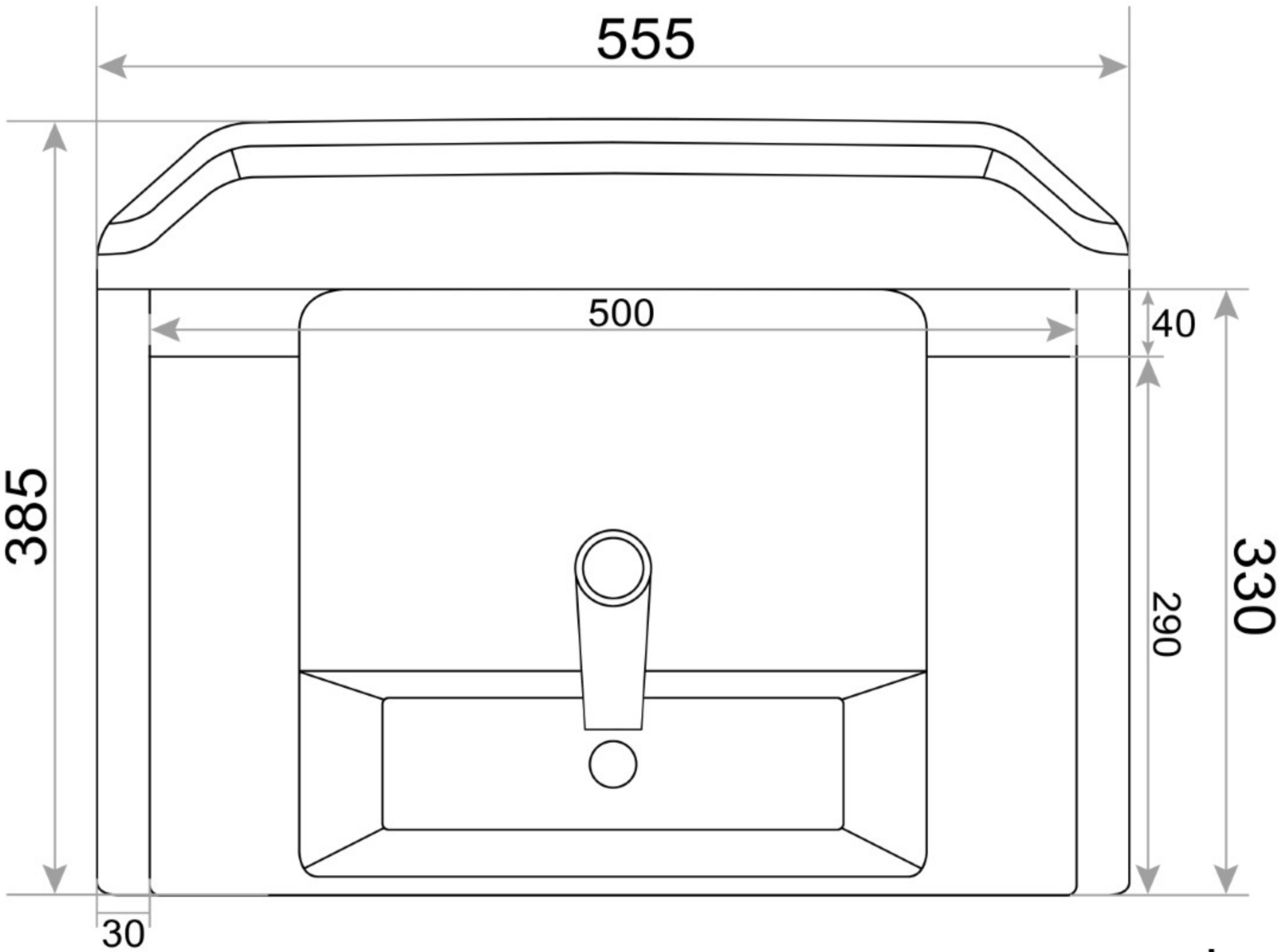
Achteraanzicht
